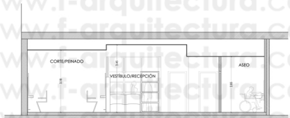
SECCIÓN_S3
