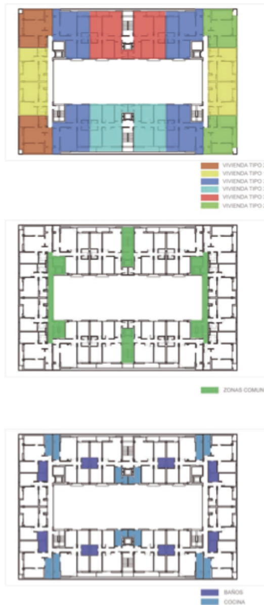
PLANTA TIPO
