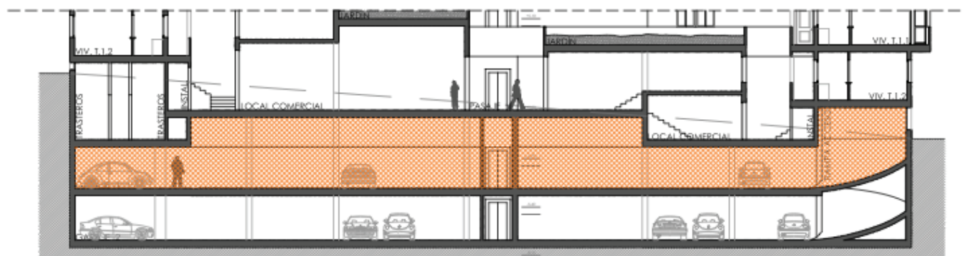
PLANTA SOTANO I
