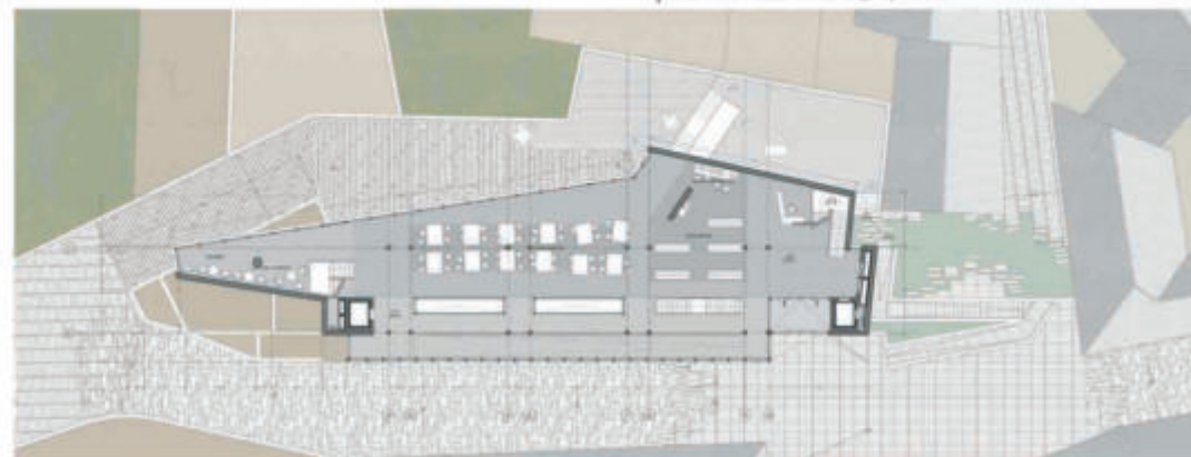
planta segunda [acceso]_1/300
