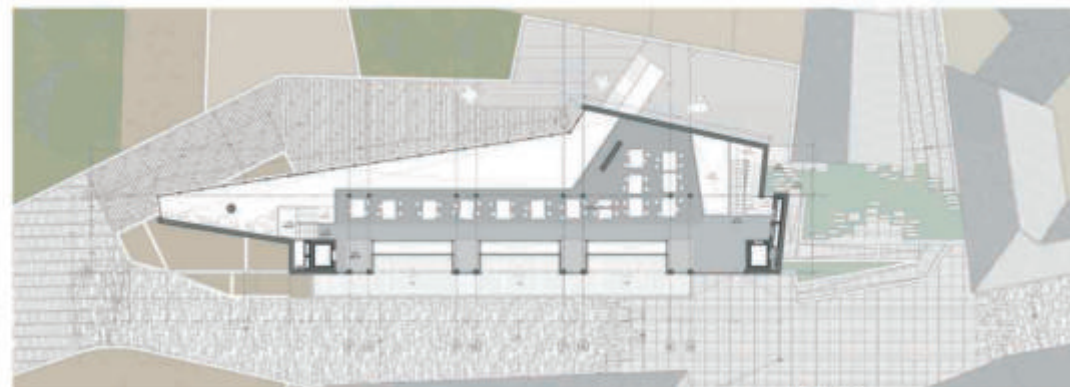
planta tercera_1/300
