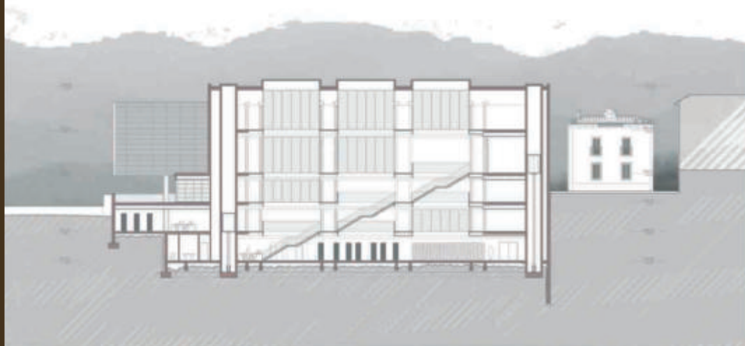
sección longitudinal_1/300
